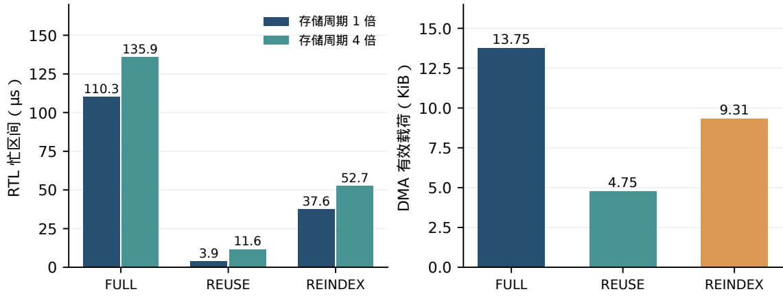
图 6: 两种在线存储周期下 H32/N64/K8 命令的实测延迟, 以及两种周期下相同的 DMA 有效载荷。REUSE 保留已有选择, REINDEX 对外部提供的候选子集重新算分; 两者工作内容不同, 不能作为可互换的精度基线。有效载荷包含结果记录与聚集 KV 数据的写回, 不含主机上传、MMIO、回读及链路封装开销。
