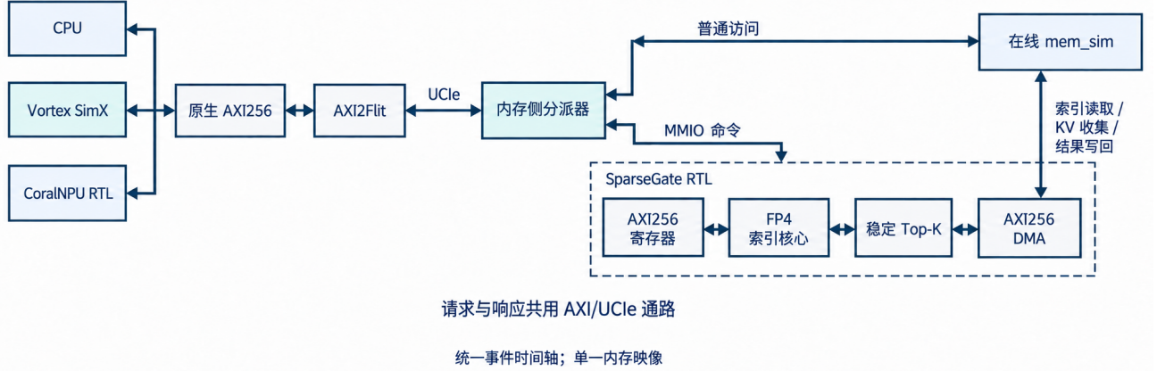
图 1: SparseGate 在统一系统中的部署位置。门控电路位于 UCle 之后，普通访问保留旁路。存储侧 C++ 分发器是验证适配层；寄存器端点、评分与选择核心以及 DMA 均由可综合 RTL 实现。返回数据与完成状态沿原有协议路径传递。本图为架构示意，精确的协议约定见配套仓库。
