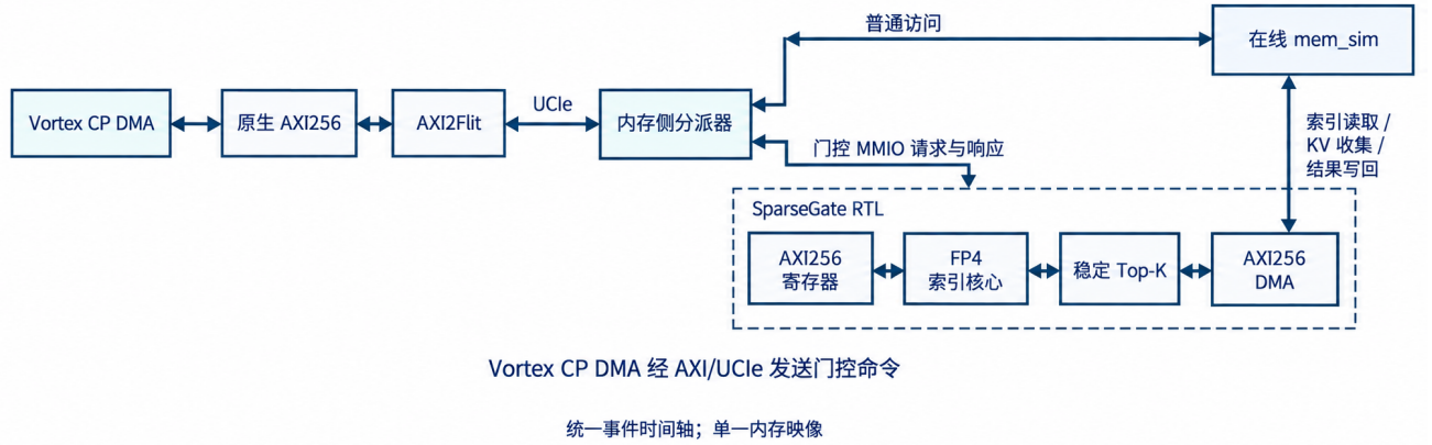
图 1: 已验证的 Vortex CP DMA 命令路径。门控 MMIO 经 AXI / UCle 到达 C++ 验证分发器与可综合的 SparseGate RTL。RTL DMA 与普通访问共用在线 mem_sim，响应沿原链路返回。图中省略 CPU 与 CoralNPU 的普通访存流量。
