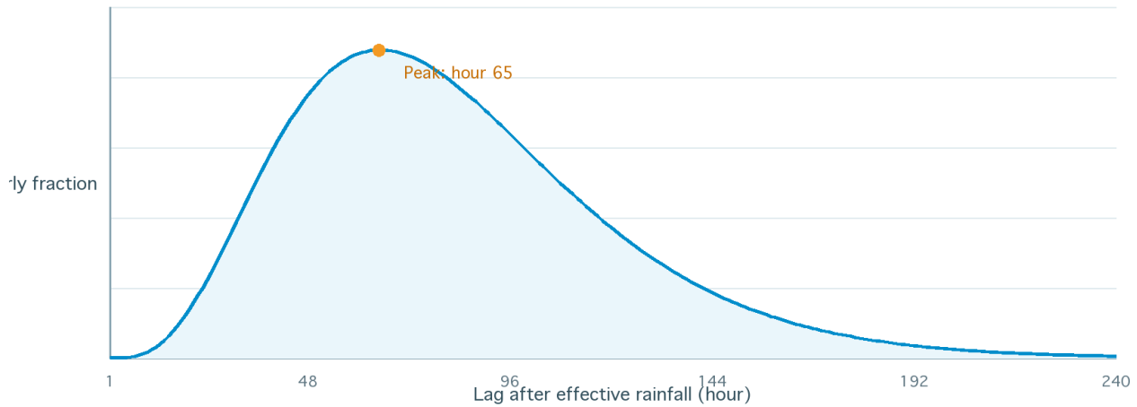
รูปที่ 2 สัดส่วนปริมาตรรายชั่วโมงของ Unit Hydrograph X.90 (ผลรวม \approx 1 )
