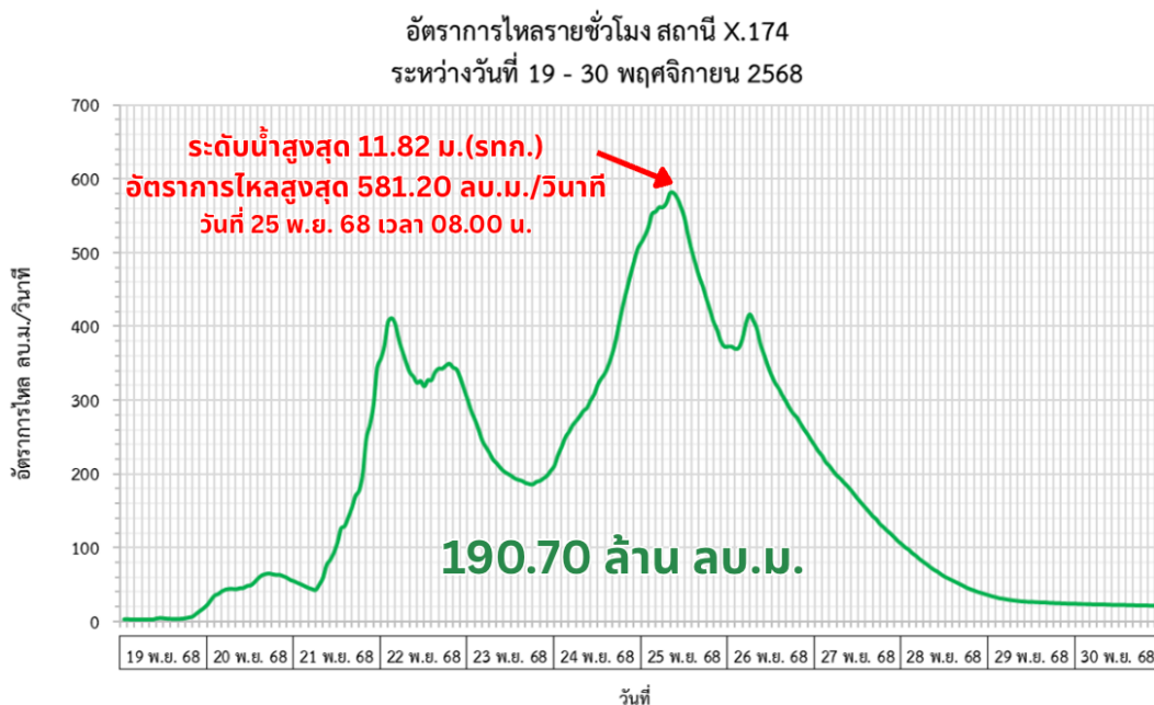
รูปที่ 4 Hydrograph ตรวจวัดสถานี X.174 ระหว่างวันที่ 19–30 พฤศจิกายน 2568
