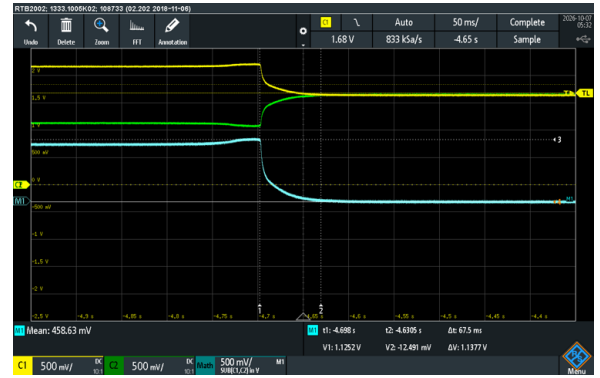
(d) Sample 2: Positive Saturation Recovery
