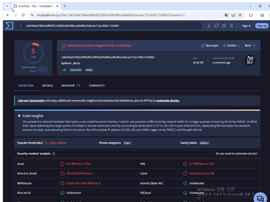
그림 2. VirusTotal 해시 기반 분석 결과 (1)
