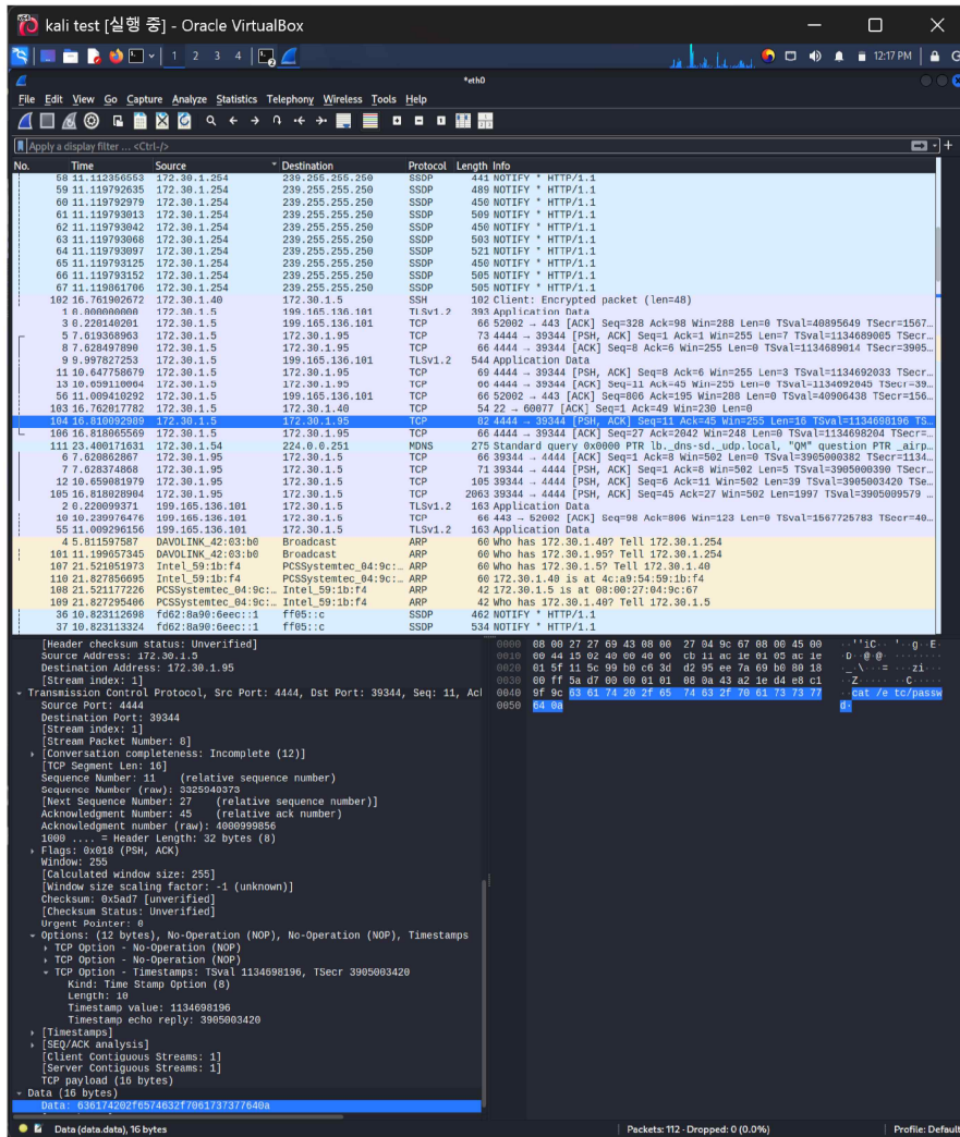
그림 20. 패킷 상세 뷰 — 리버스셸 세션 TCP 페이로드에서 "cat /etc/passwd" 명령 데이터 확인
