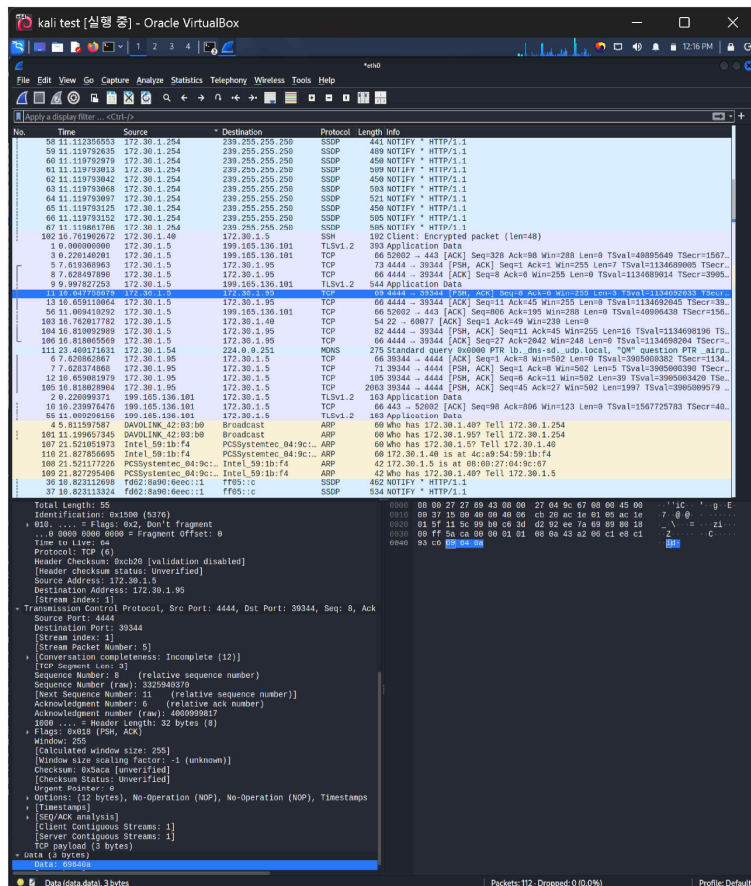
그림 19. 패킷 상세 뷰 — 리버스셸 세션 TCP 페이로드에서 "id" 명령 데이터 확인
