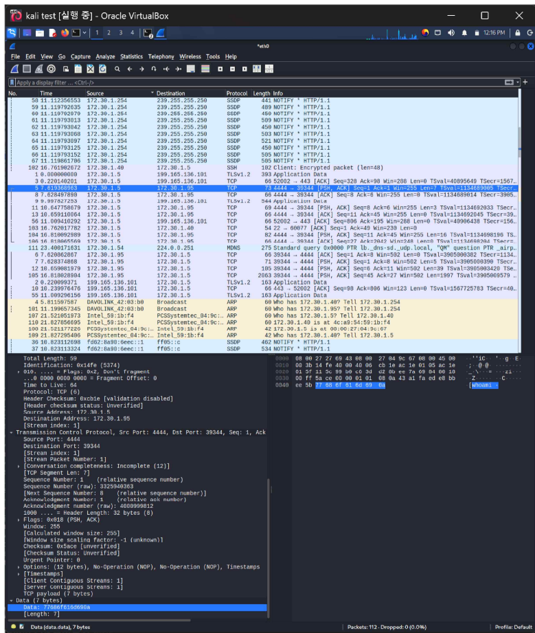
그림 18. 패킷 상세 뷰 — 리버스셸 세션 TCP 페이로드에서 "whoami" 명령 데이터 확인
