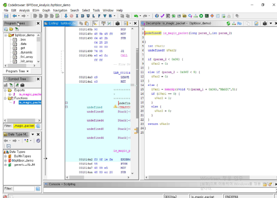
그림 16. Ghidra를 이용한 is_magic_packet() 함수 분석
