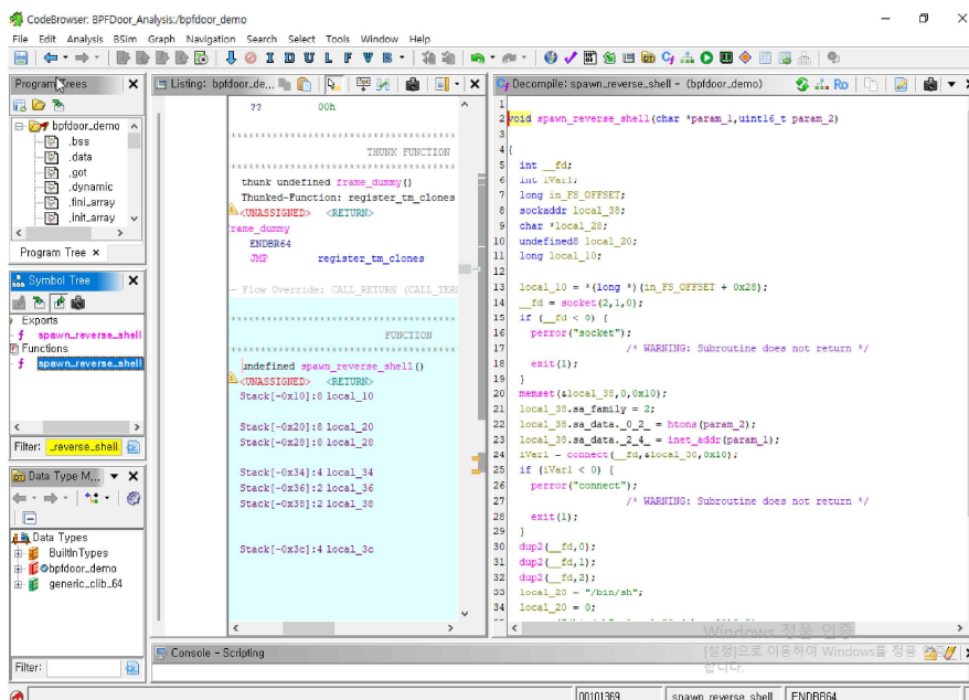
그림 14. Ghidra를 이용한 spawn_reverse_shell() 함수 분석 (1)
