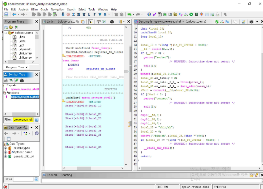
그림 15. Ghidra를 이용한 spawn_reverse_shell() 함수 분석 (2)
