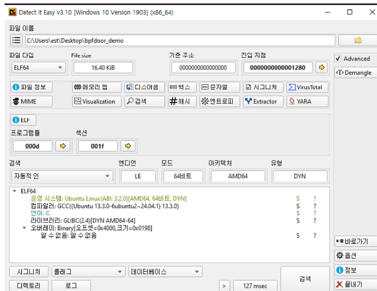
그림 5. Detect It Easy를 이용한 실행파일 분석 결과
