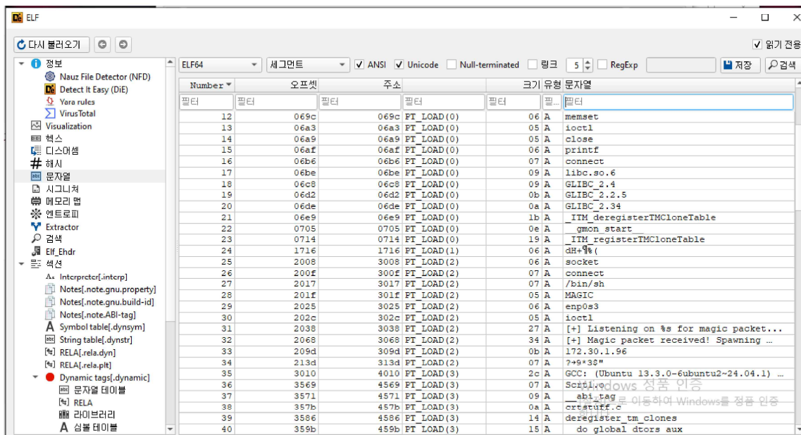
그림 8. Detect It Easy(DiE)를 이용한 실행 파일 문자열 분석
