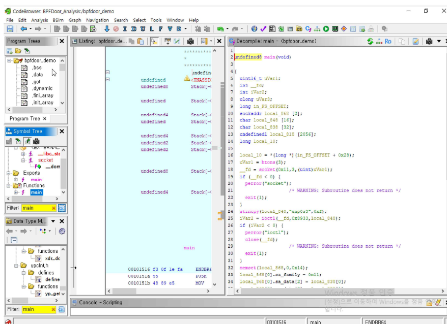
그림 12. Ghidra를 이용한 main() 함수 분석 (1)
