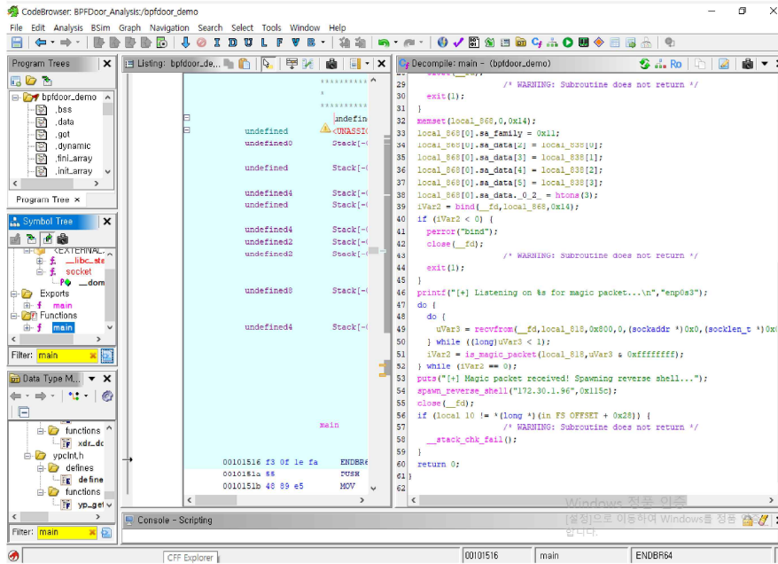
그림 13. Ghidra를 이용한 main() 함수 분석 (2)
