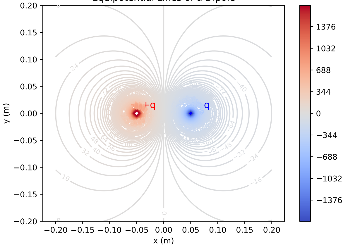
Equipotential Lines of a Dipole
