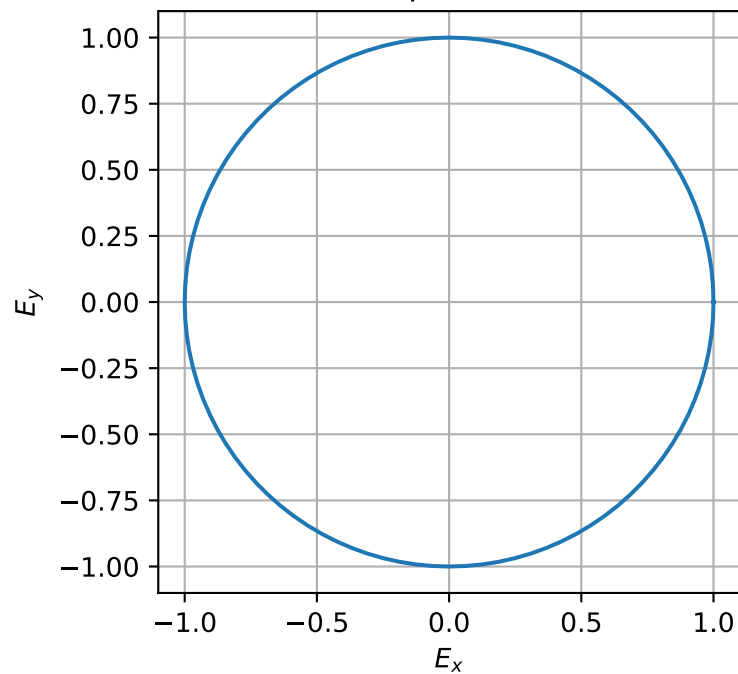
\Delta\phi = \pi/2
