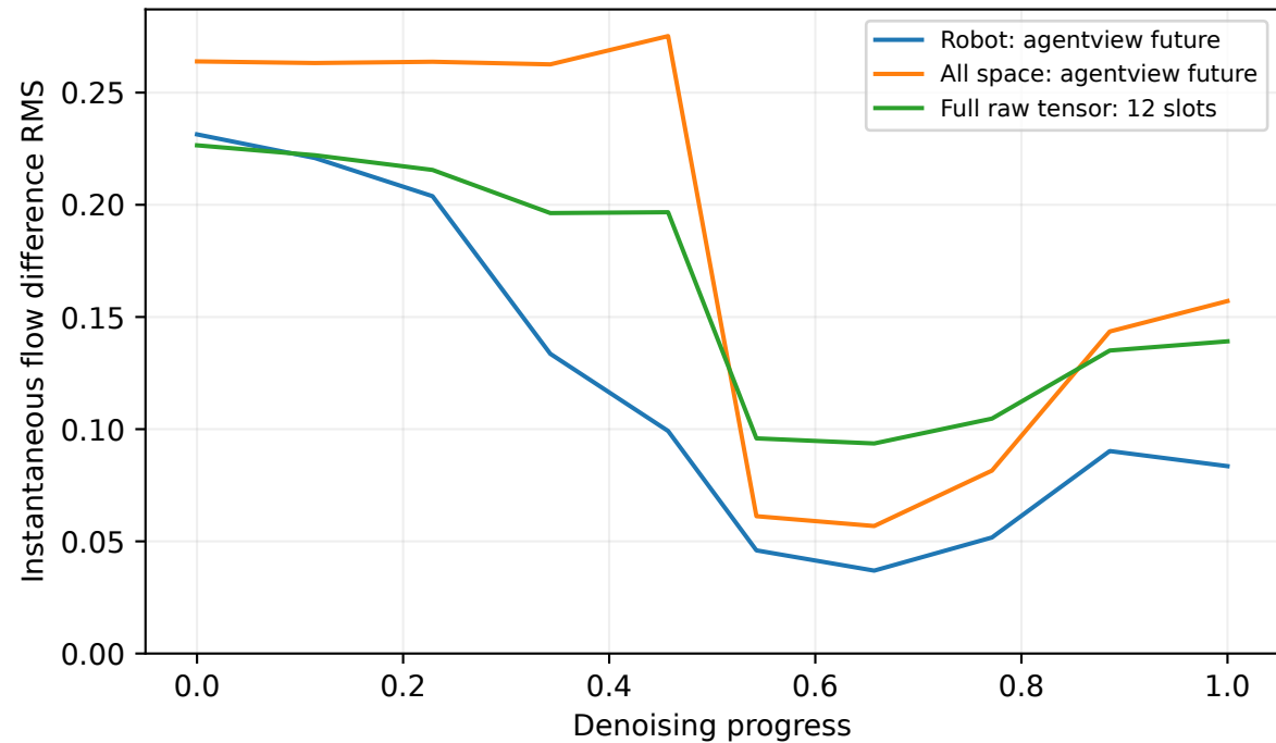
T05 · BG8 vs BG0 · seed 0
