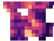
L5 · frames17-20
