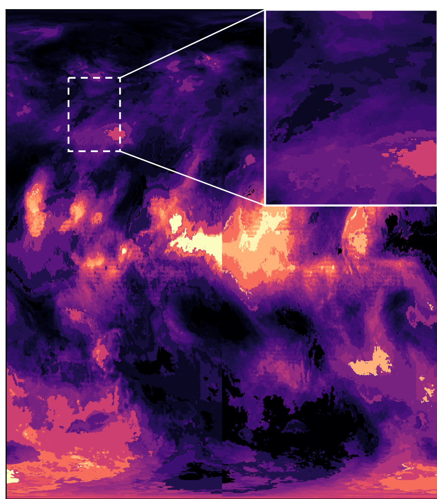
(d) cuZFP (CR=16.0, PSNR=21.51 dB, SSIM=0.720)
