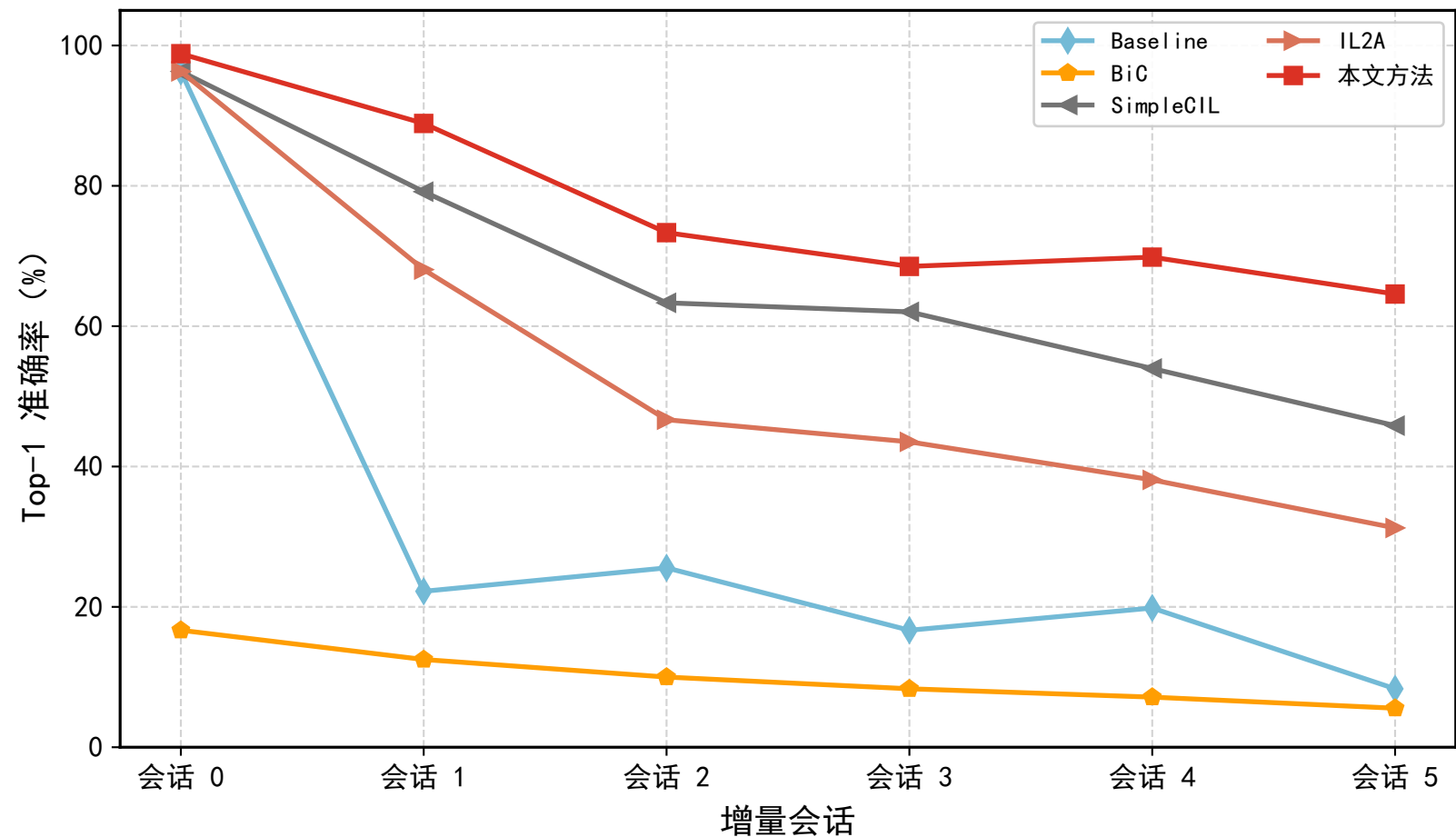
WiAR (16 类) 类增量各会话准确率
