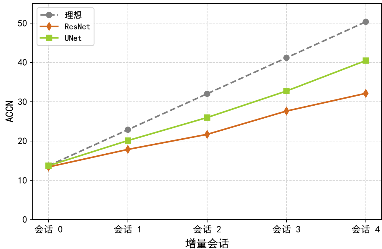
不同骨干网络的 ACCN
