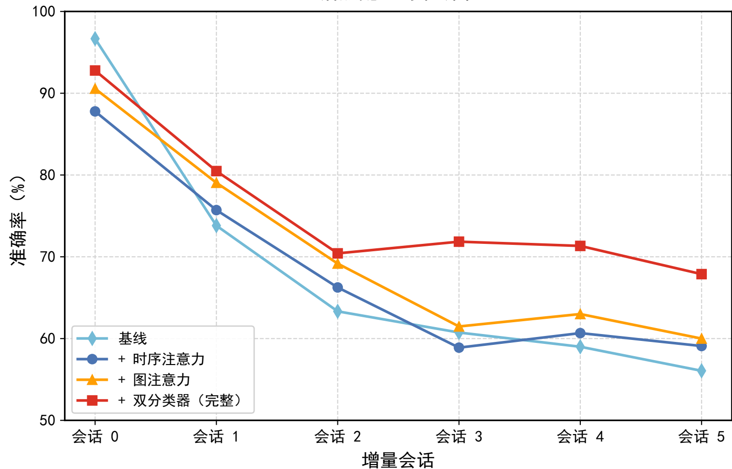
消融配置的准确率
