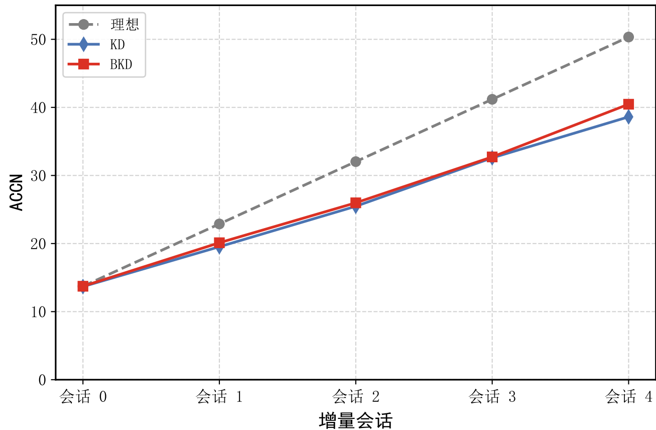
KD 与 BKD 的 ACCN 对比
