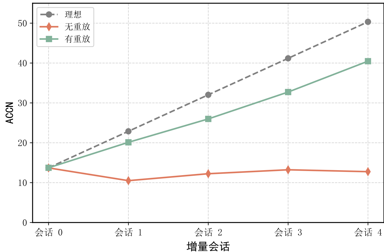
有无样本重放的 ACCN
