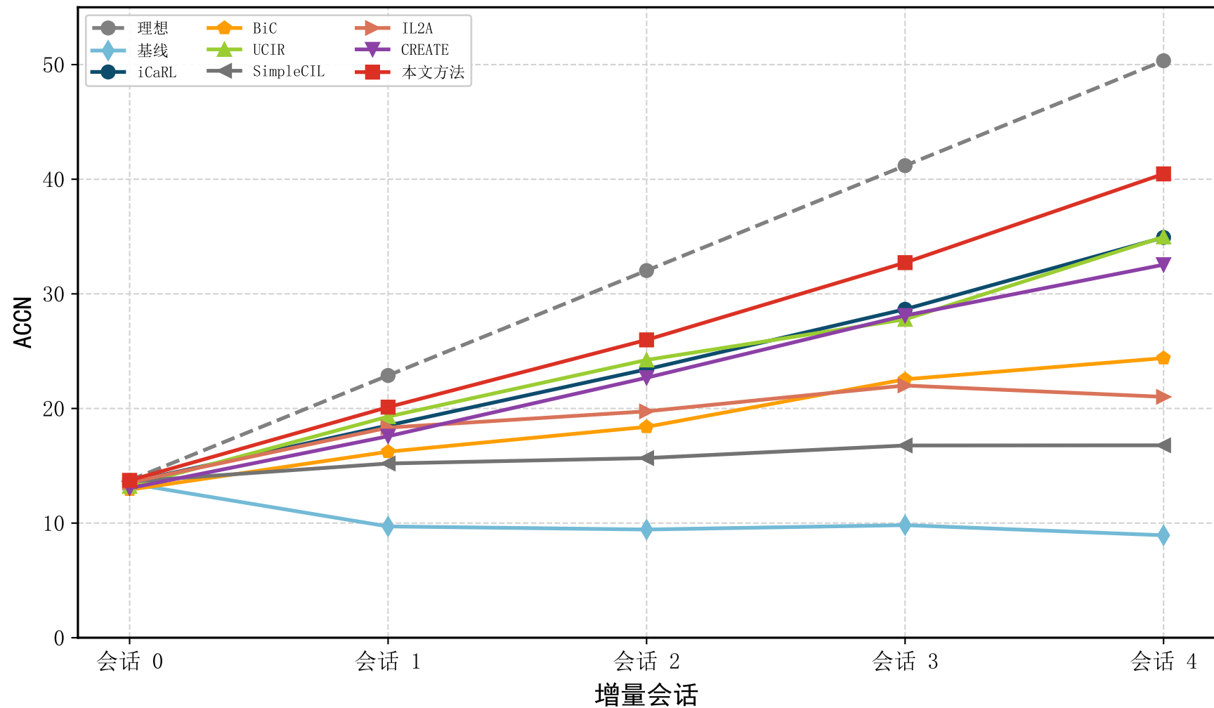
不同类增量学习方法的 ACCN
