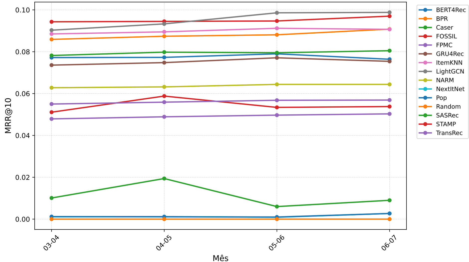
Variação Mensal do MRR@10 (Ranking Completo)
