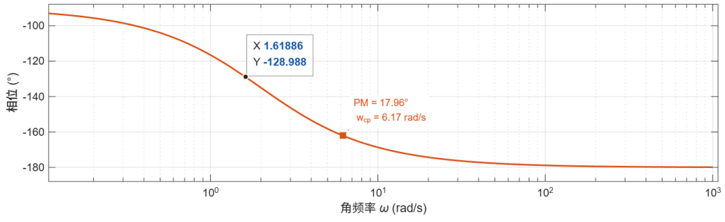
图 2.7. 原系统的相频曲线
