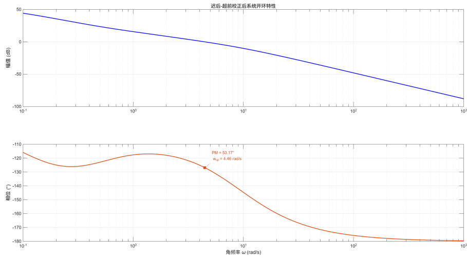
图 2.5. 校正后系统伯德图
