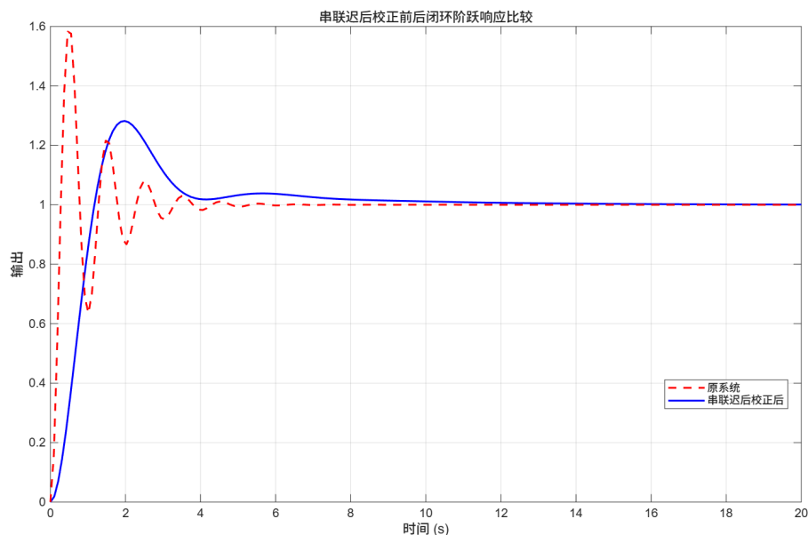
图 2.11. 校正后系统阶跃响应
