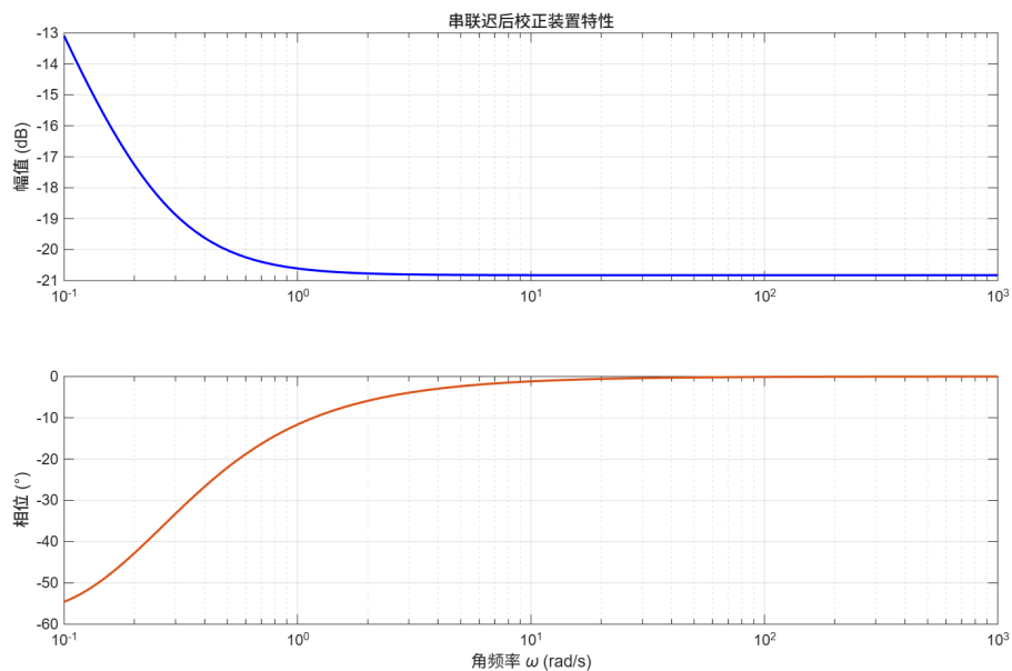
图 2.9. 校正装置伯德图
