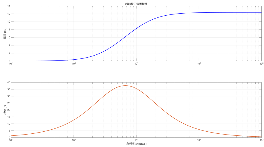
图 2.1. 校正装置伯德图
