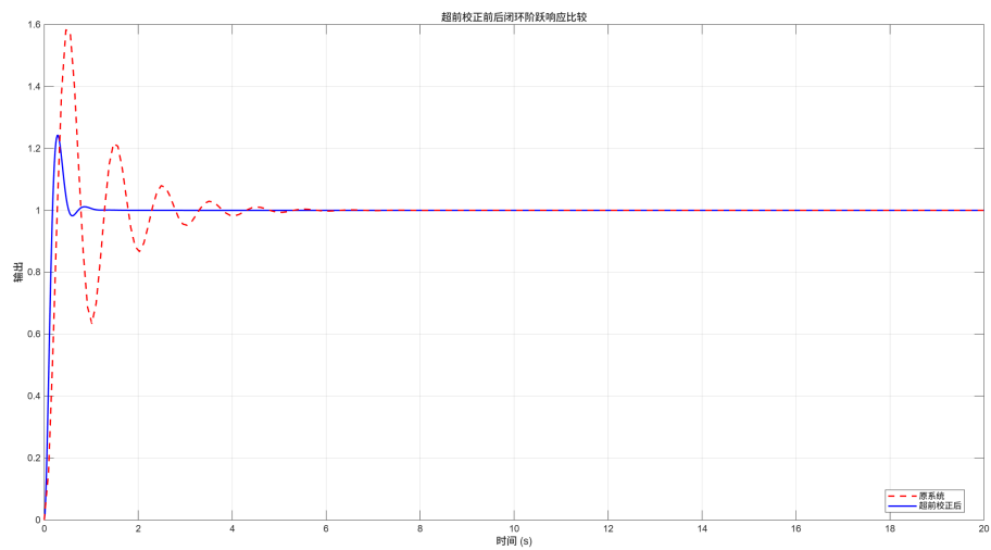
图 2.3. 校正后系统阶跃响应
