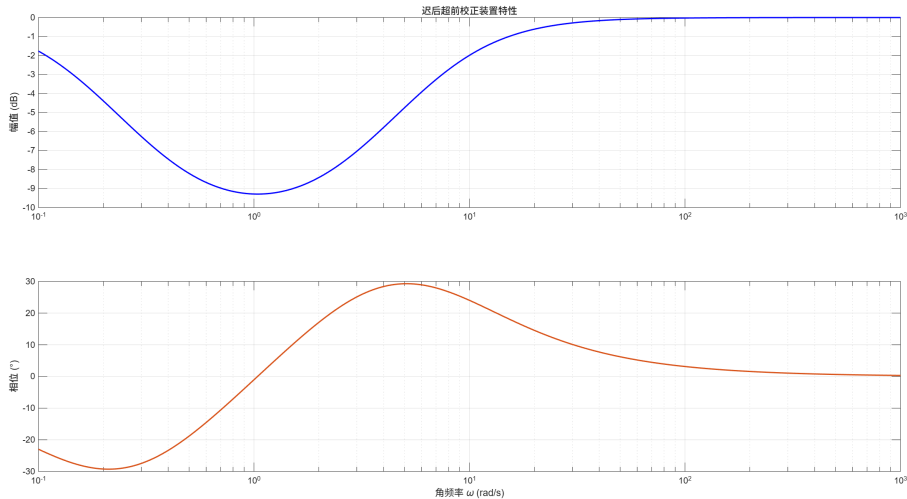
图 2.4. 校正装置伯德图
