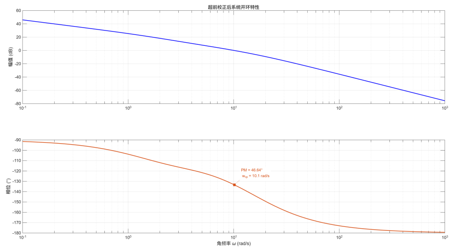
图 2.2. 校正后系统伯德图
