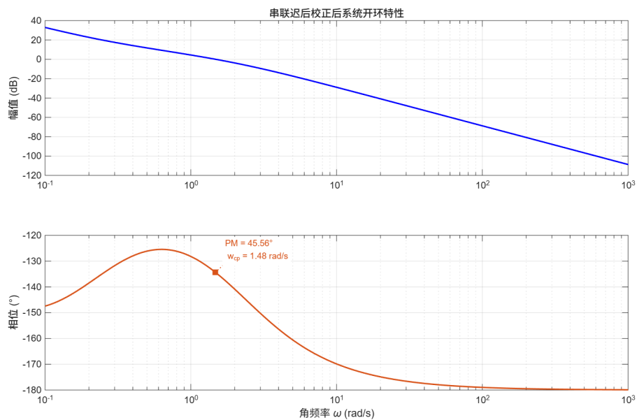
图 2.10. 校正后系统伯德图
