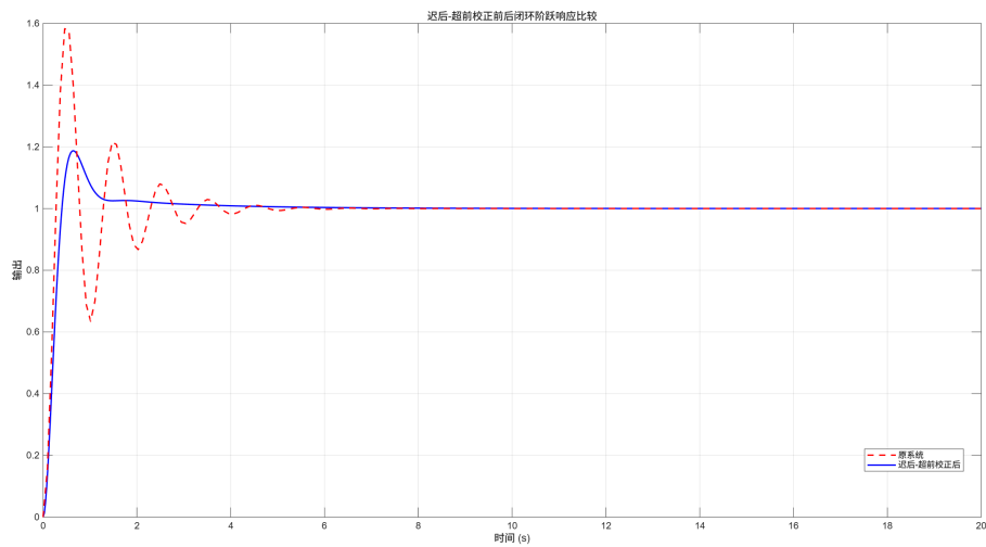
图 2.6. 校正后系统阶跃响应
