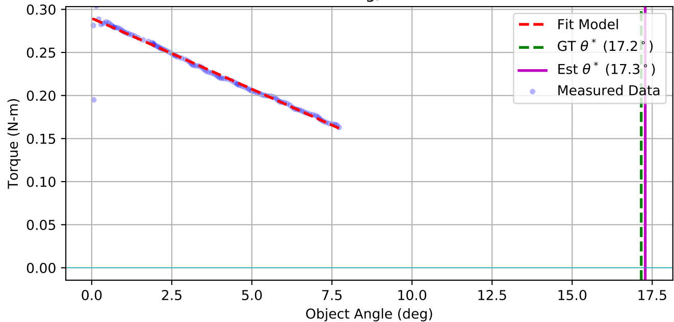
Fit: m=0.65\text{kg} , z_c=0.145\text{m}
