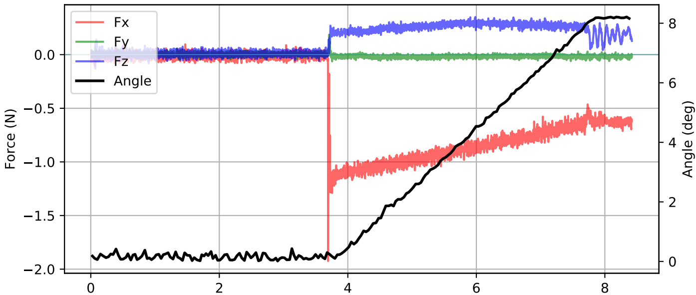
Fit: m=0.65\text{kg} , z_c=0.145\text{m}
