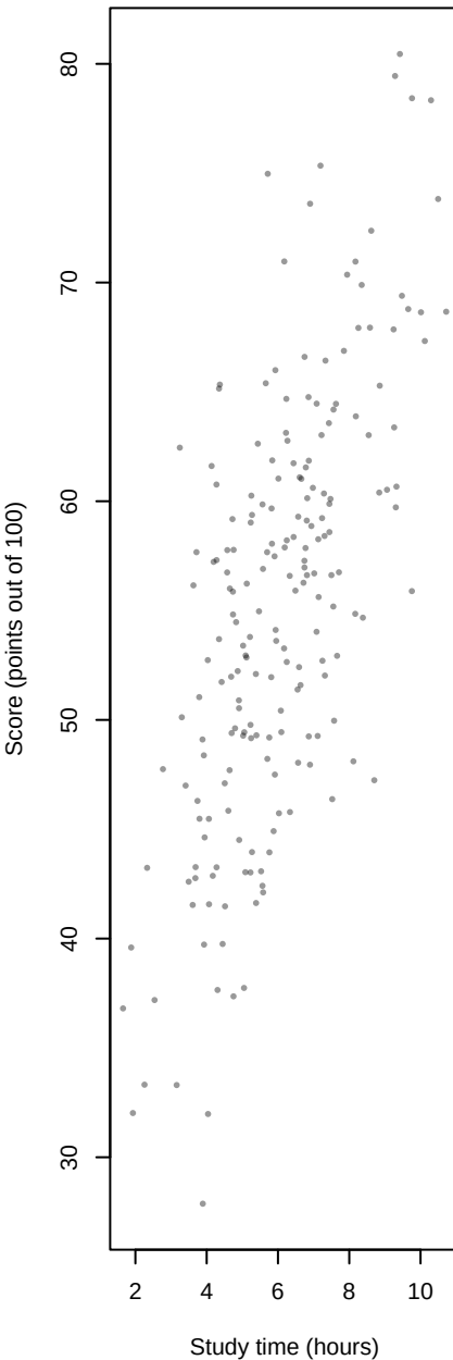
Cov = 12.2
