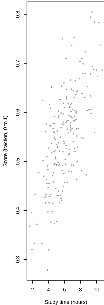
Cov = 0.122
