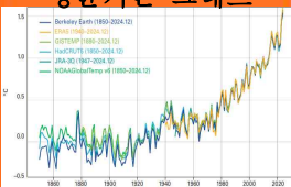
1850년~2024년 지구 평균기온 그래프
