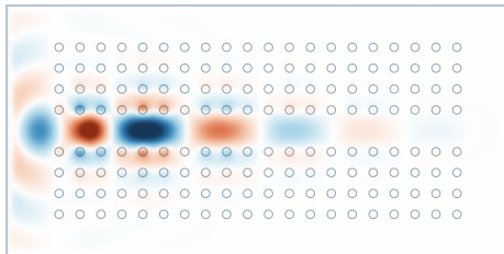
E_z , step 4200
