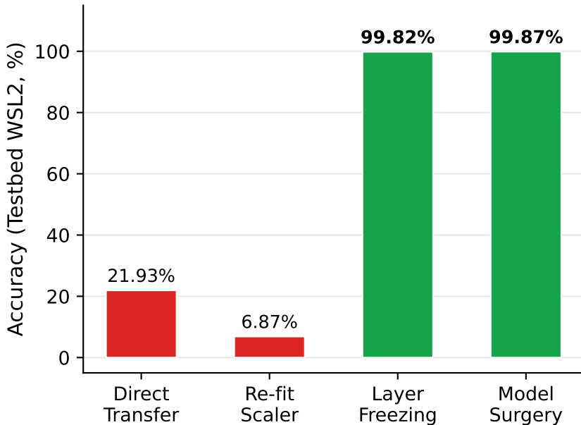
Accuracy qua các can thiệp
