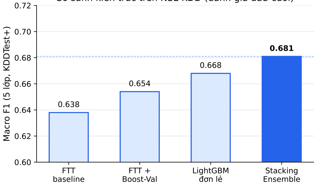
So sánh kiến trúc trên NSL-KDD (đánh giá đầu-cuối)
