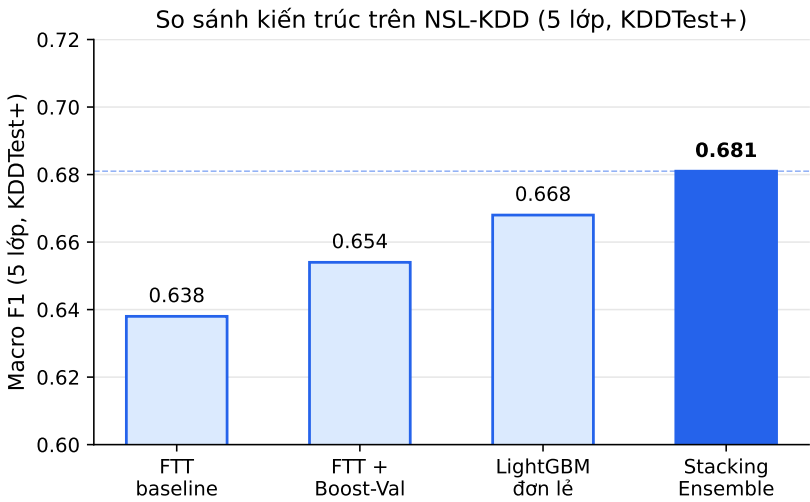
Hình 5.1: So sánh Macro F1 qua các phiên bản kiến trúc trên NSL-KDD (5 lớp, KDDTest+).
