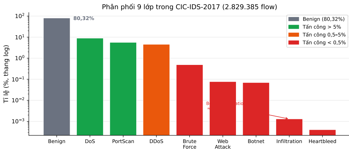
Hình 3.2: Phân phối lớp trong CIC-IDS-2017 (2.829.385 flow, thang logarithm). Benign chiếm 80,32%; tỉ lệ Benign:Infiltration khoảng 63.100:1.
