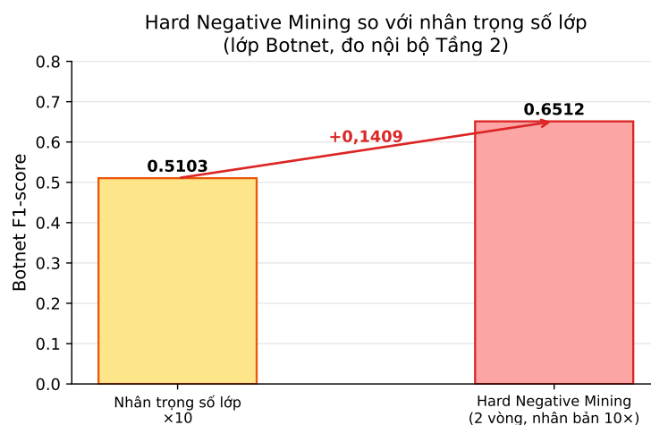
Hình 5.3: So sánh hiệu quả của Hard Negative Mining và nhân trọng số lớp trên lớp Botnet.
