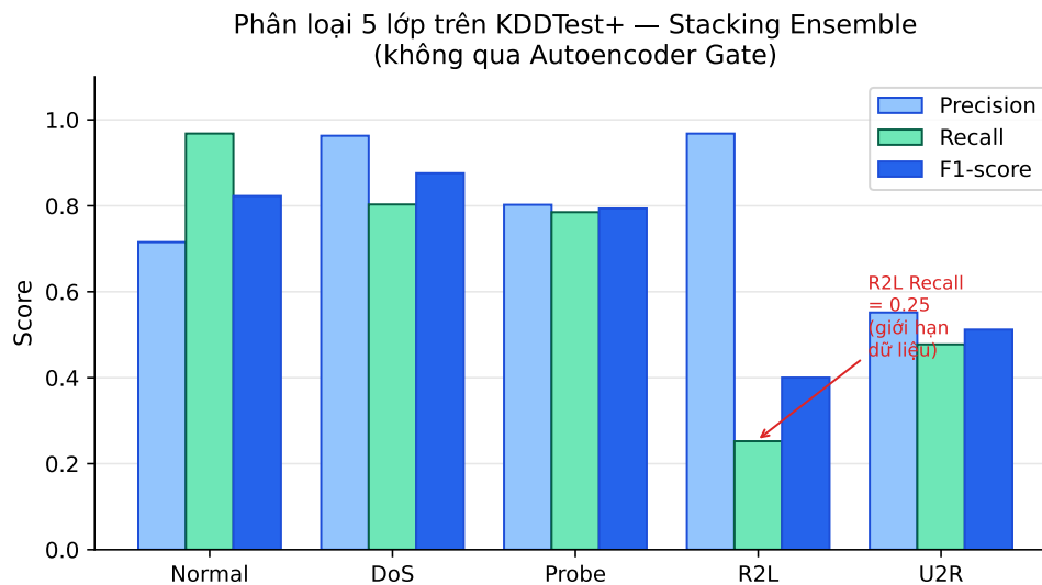
Hình 5.2: Kết quả phân loại 5 lớp trên KDDTest+ — Stacking Ensemble (FTT + LightGBM → Meta-LR).
