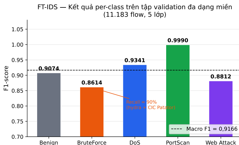
Hình 5.7: FT-IDS — F1-score per-class trên tập validation đa dạng miền (11.183 flows). Đường ngang thể hiện Macro F1 = 0,917.
