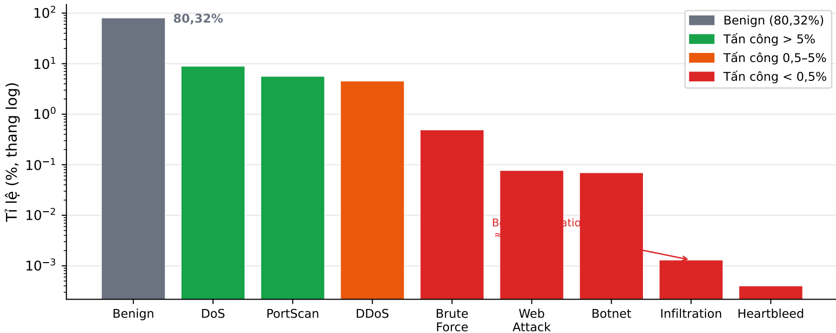
Phân phối 9 lớp trong CIC-IDS-2017 (2.829.385 flow)
