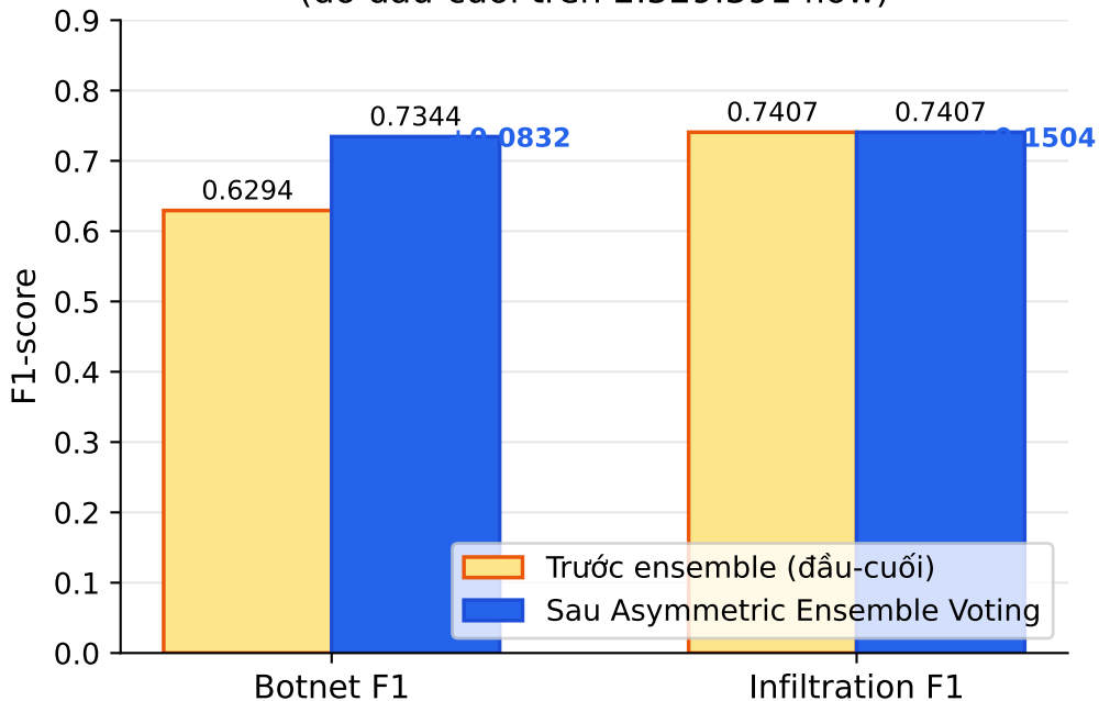
Đóng góp của Asymmetric Ensemble Voting (đo đầu-cuối trên 2.529.391 flow)
