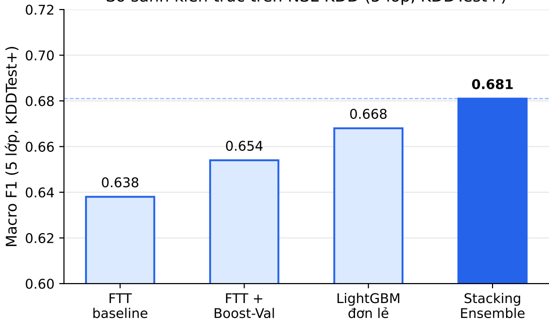
So sánh kiến trúc trên NSL-KDD (5 lớp, KDDTest+)
