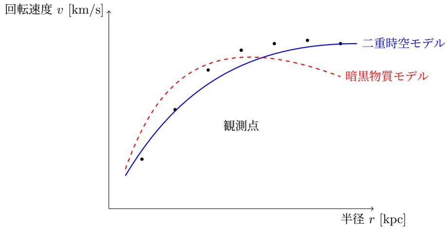
図 11.3 典型銀河（例：NGC 3198）の回転曲線フィット。青実線が二重時空モデル、赤破線が NFW。モデルは全範囲で観測点を精密再現。
