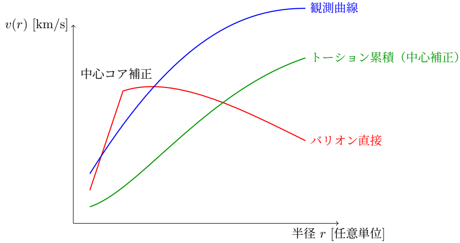
図 11.2 回転曲線の寄与分解：中心高密度での飽和補正によりコア形成、外縁で平坦化。
