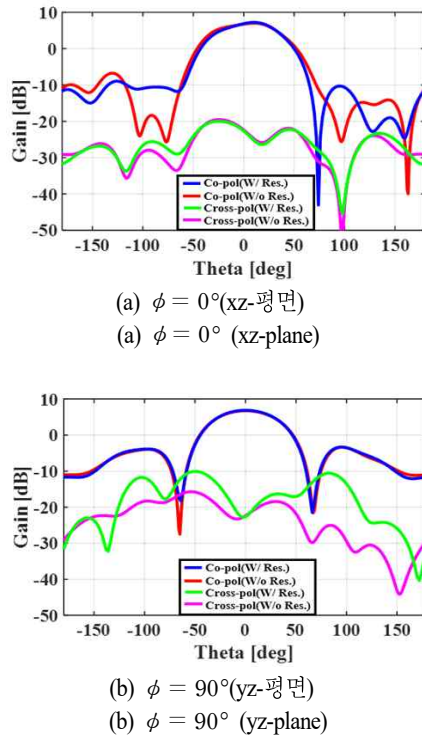
그림 13. 공진기 유무에 따른 안테나의 방사패턴 모의실험 결과
