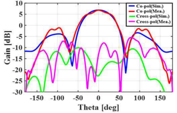
(b) \phi = 90^\circ (yz-plane)
