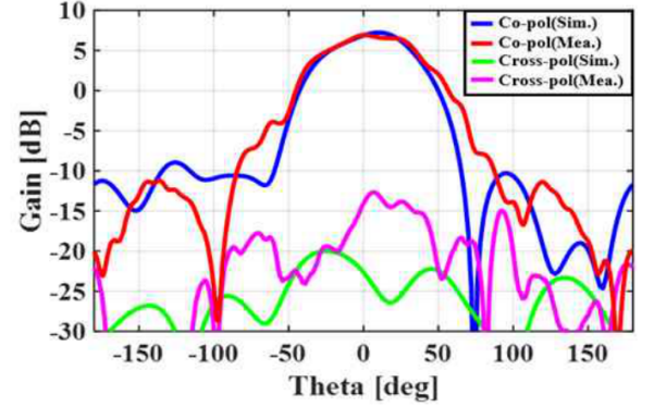
(a) \phi = 0^\circ (xz-plane)
