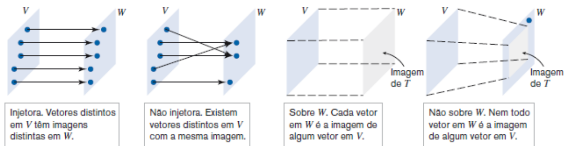
Figura 11 – Diagrama do isomorfismo e sua imagem (NADA, e), pg. 445.
