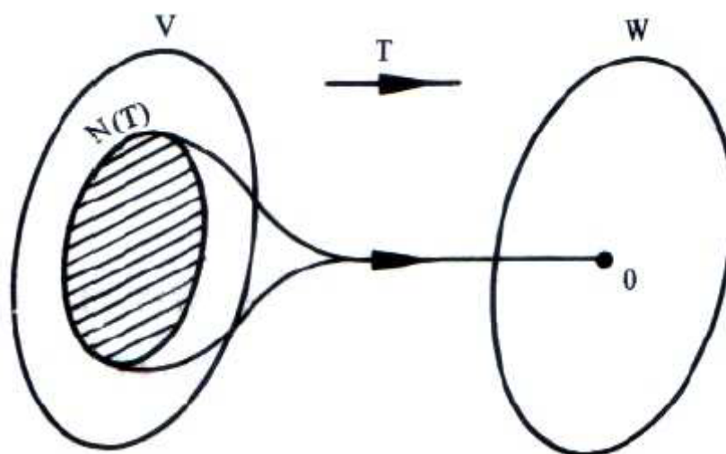
Figura 9 – Diagrama do núcleo de uma transformação linear (NADA, d).
