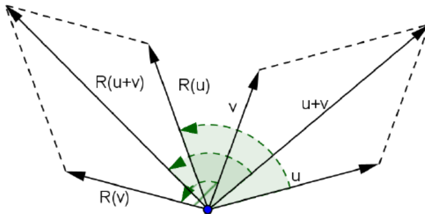
Figura 8 – Transformada de rotação de um vetor (NADA, c).
