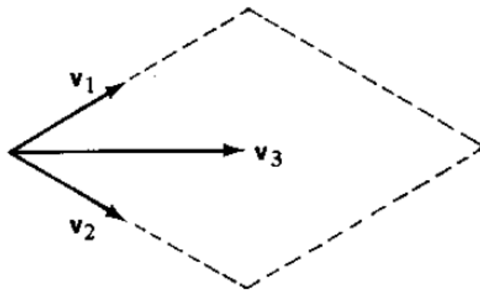
Figura 4 – Combinação de três vetores lineares (NADA, a), pg. 113.
