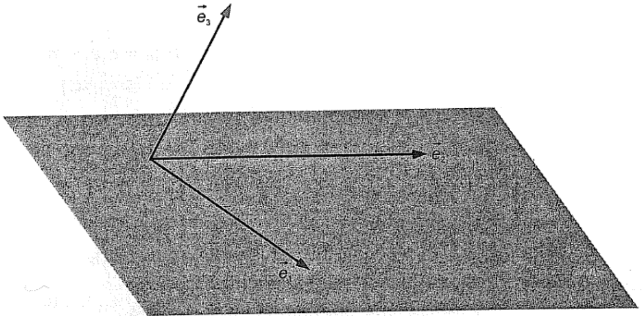
Figura 6 – Base de um vetor em \mathbb{R}^3 (NADA, b), pg. 52.
