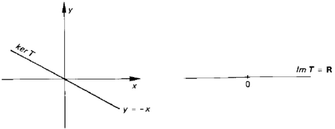
Figura 10 – Imagem de um núcleo de transformação linear (NADA, a), pg. 152.
