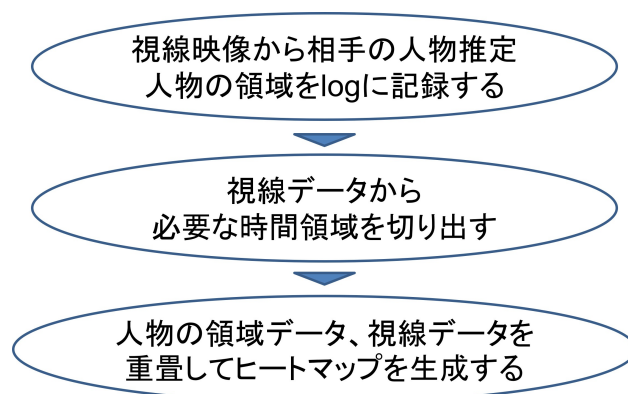
図 4.4 YOLO11 を用いたヒートマップ生成フロー
