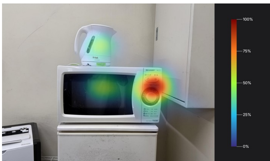
図 4.2 静止物体に対する生成成功例
