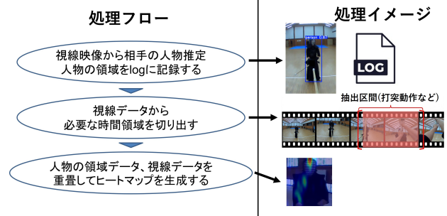
図 2 YOLO11 を用いたヒートマップ生成フロー
