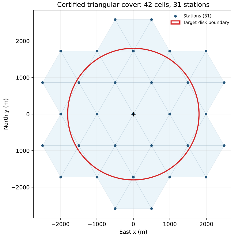
图 4 边长 995 m 的定向源三角网格覆盖基线（42 个三角形、31 个检测点）
