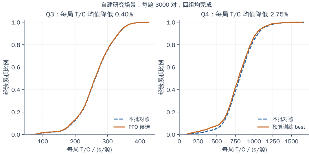
图 5 问题三、四最新配对批次的逐场景每源耗时经验分布；曲线越靠左表示在相同比例的场景上耗时越低
