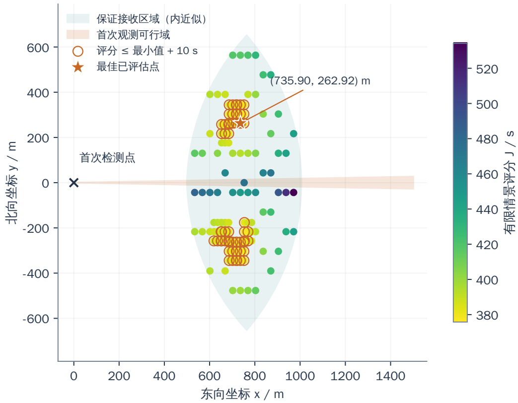
图 2 保证接收区域内的有限候选评分；星号为综合代价最小的已评估点，颜色不代表连续域全局最优性
