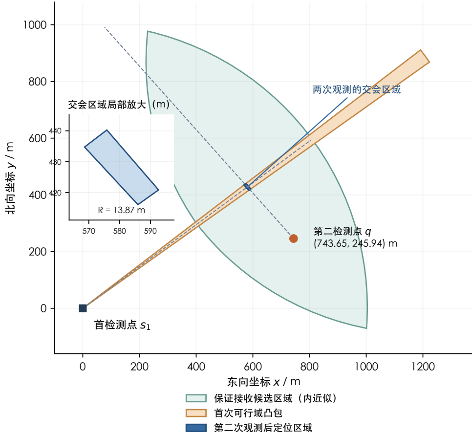
图2 同一构造场景中的第二检测点与交会定位结果。虚线为两次实测示向线；局部放大显示补测后的定位区域。候选区域由首次可行域凸包保守构造，各坐标轴均按等比例绘制。
