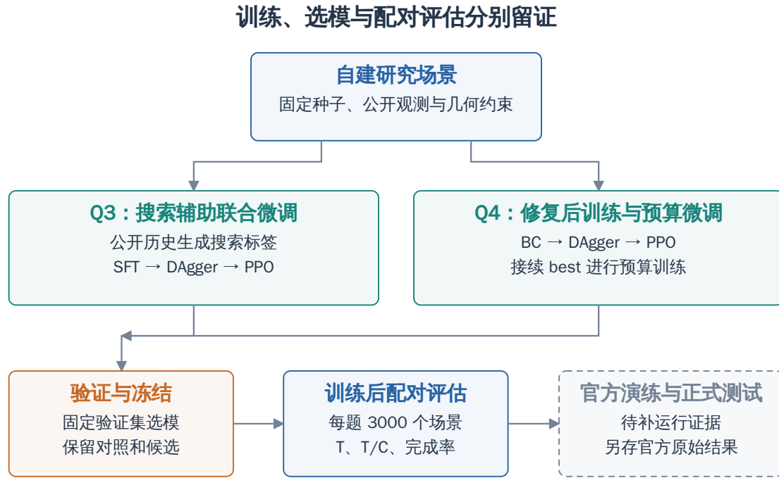
图 7 训练、验证选模与冻结后配对评估相互隔离的实验流程；官方测试为待补环节
