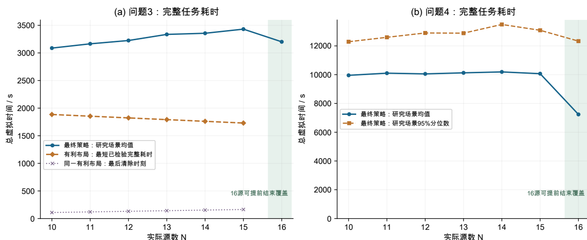
图7 最终策略在全部清除并取得退出依据条件下的耗时。问题三：研究场景均值与同一最终模型的有利布局对照，布局曲线为有限候选实测值；问题四：研究场景均值及95%分位数。各曲线的总耗时均包含无遗漏确认。
