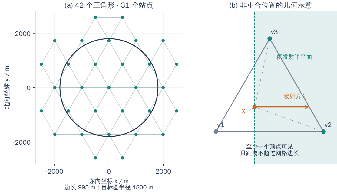
图 6 边长 995 m 的三角网格以 42 个闭三角形、31 个检测点提供方向无关的发现证书
