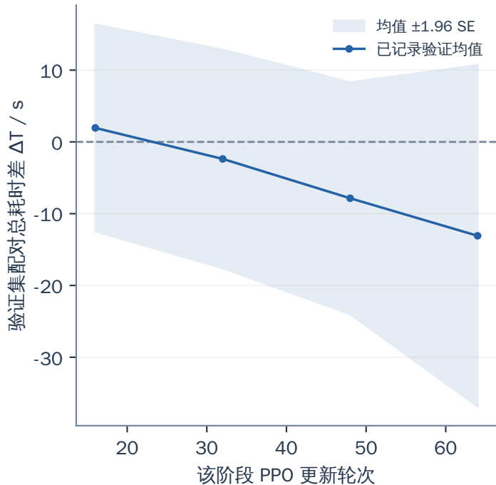
Q3 : 联合 PPO 阶段
