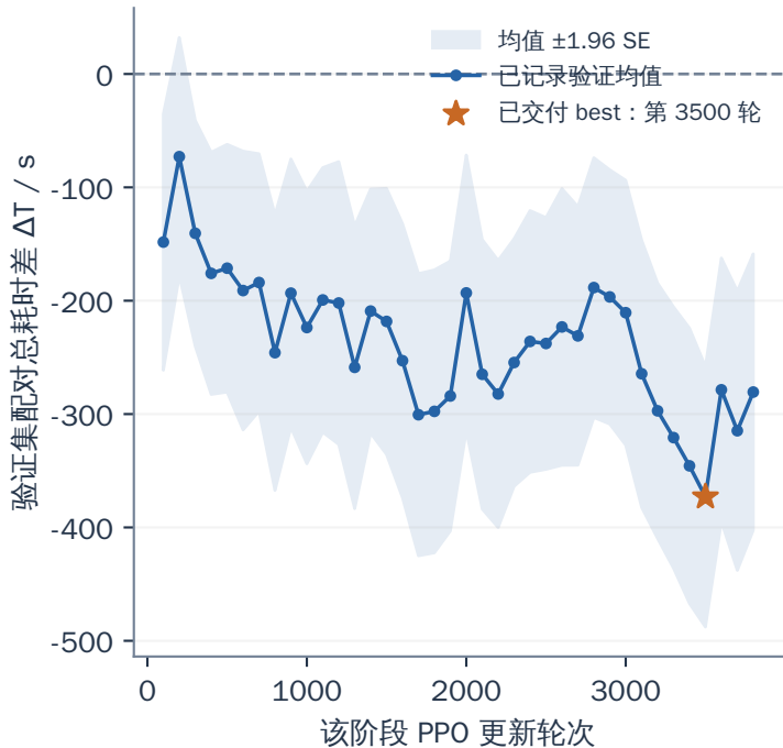
Q4 : 预算 PPO 阶段
