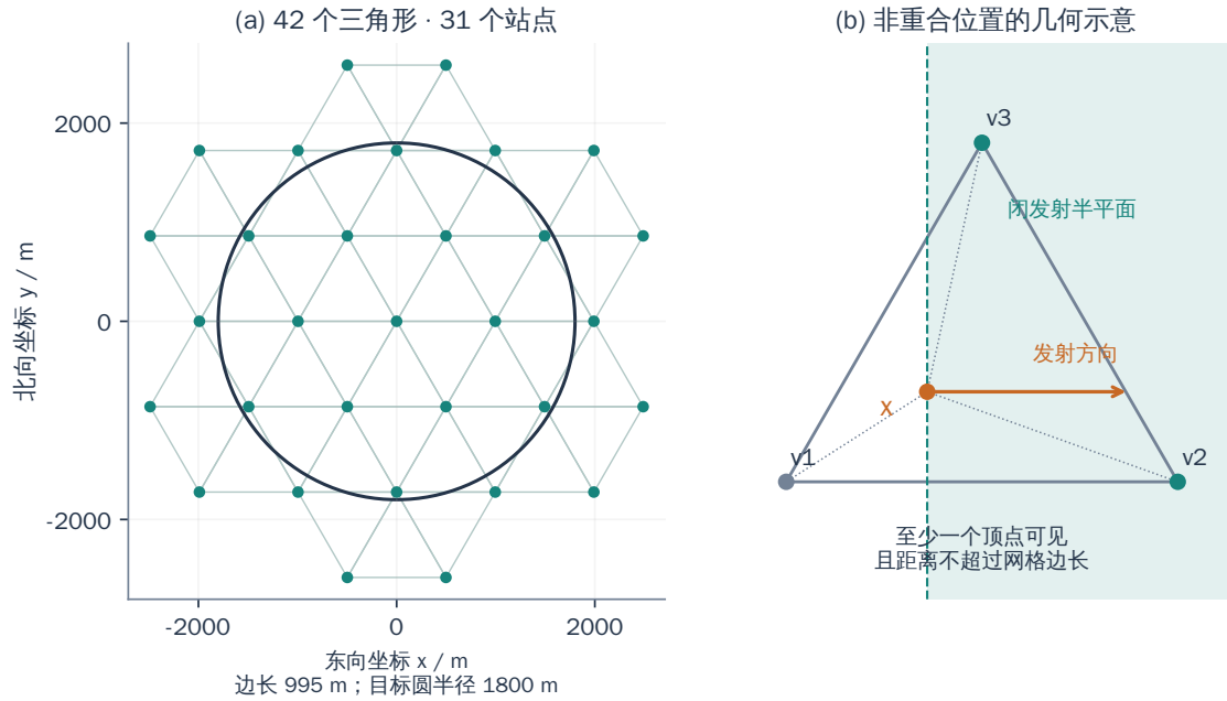
图 5 边长 995 m 的定向源三角网格覆盖基线（42 个三角形、31 个检测点）
