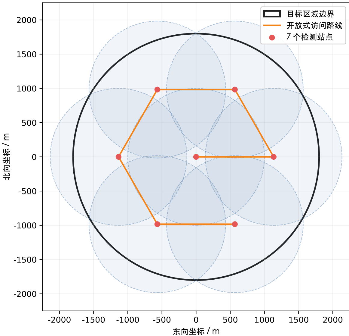
全向源七点覆盖骨架 (外圈半径 1135 m)
