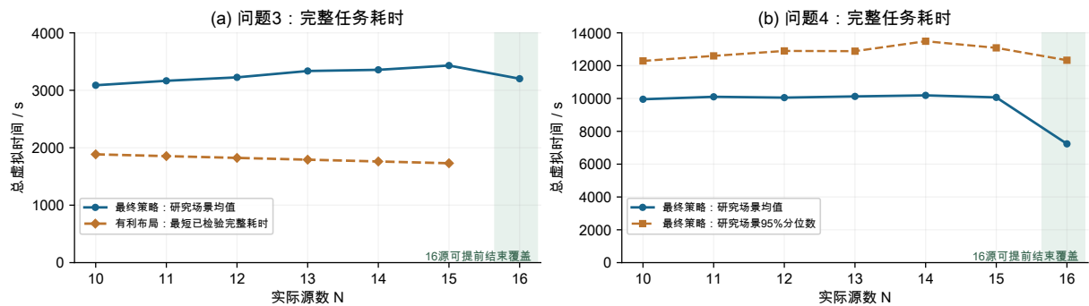
图 6 最终策略在全部清除并取得退出依据条件下的耗时。问题三：研究场景均值与同一最终模型的有利布局对照，布局曲线为有限候选实测值；问题四：研究场景均值及 95% 分位数。各曲线的总耗时均包含无遗漏确认。
