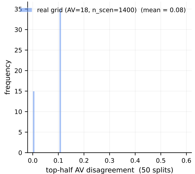
(c) Top-half AV identity shifts across subsets
