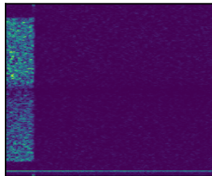
(d) Deceptive
