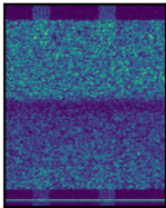
(d) Deceptive
