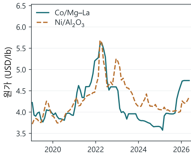
(a) 암모니아 분해
