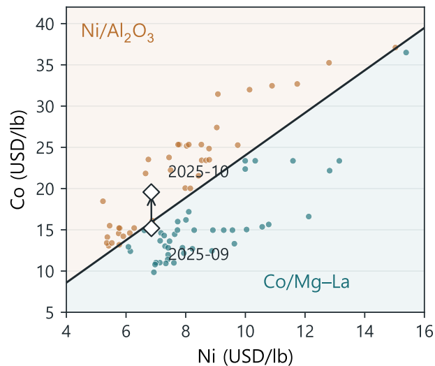
(d) 암모니아 분해 원가 경계
