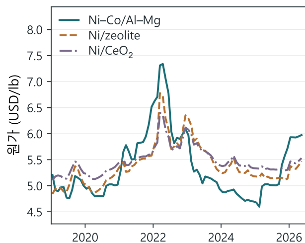
(b) 메탄 건식 개질
