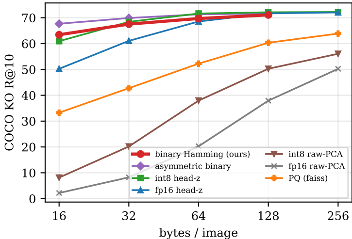
Equal-byte accuracy (KO)
